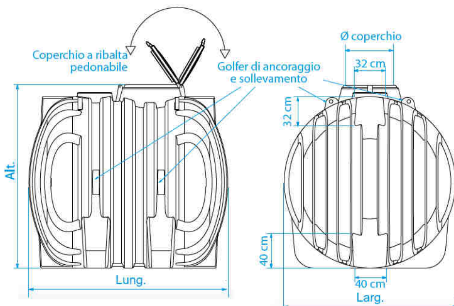
PROLUNGA MODULARE OPZIONALE (mod. PP77)
