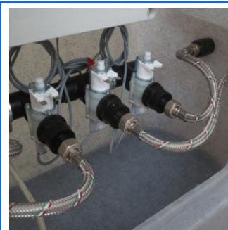
Erogazione con rubinetti da 1/2" con contaltri
